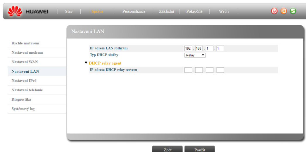
Obrázek 2-19 Nastavení LAN – relay
