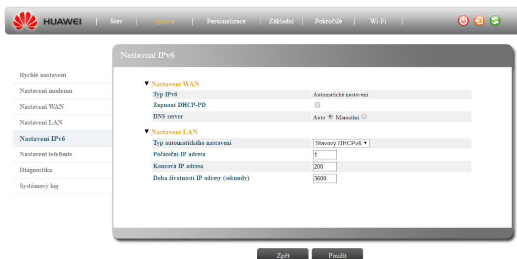
Obrázek 2-23 Nastavení IPv6 – Stavový DHCPv6
