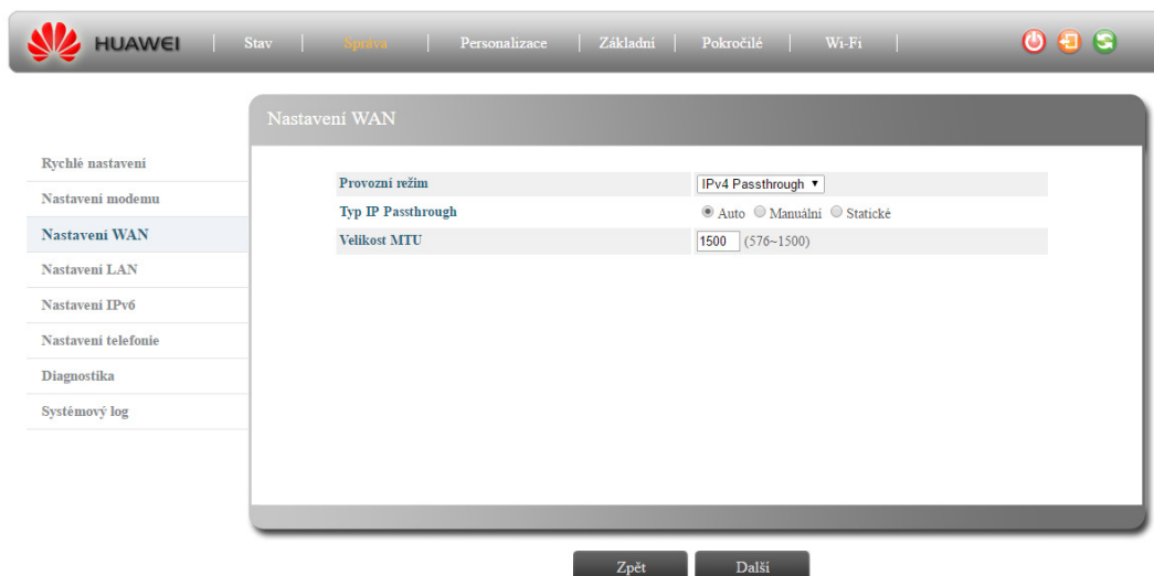
Obrázek 2-14 Nastavení WAN – IPv4 Passthrough (Auto)
