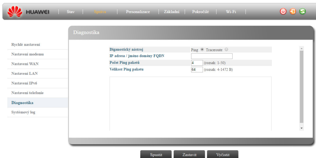
Obrázek 2-29 Diagnostika – příkaz ping
